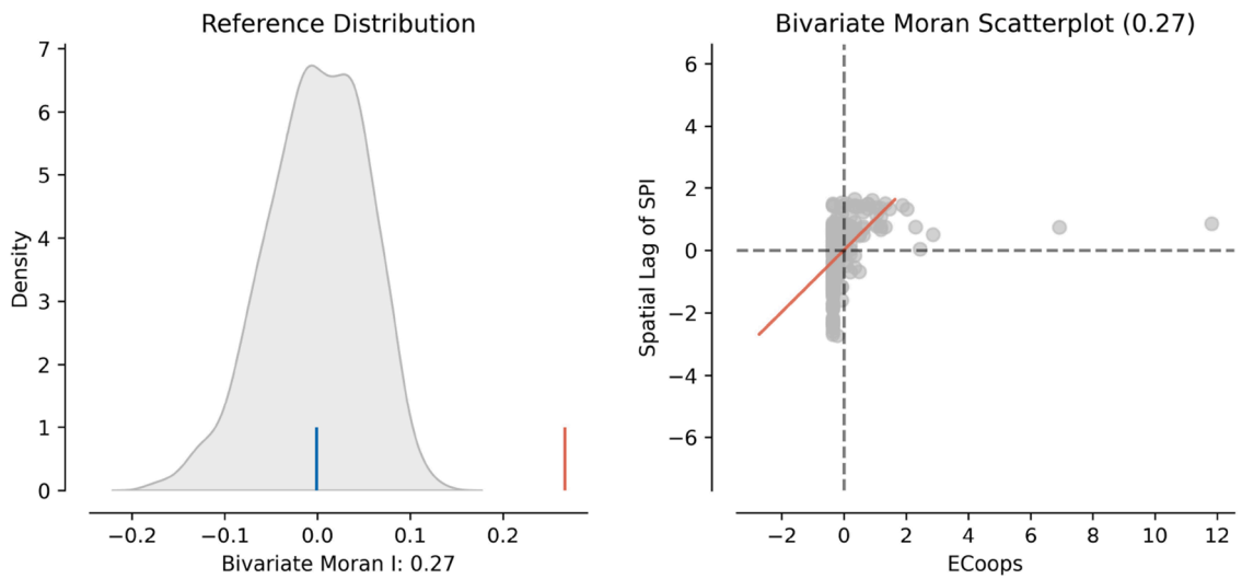
Fig. D1. Bivariate global moran statistics SPI.
