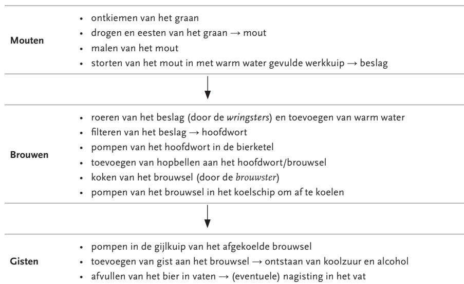
Figuur 2.1 Schematische weergave van het brouwproces
