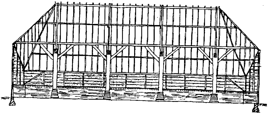
doorsnede C.D.
