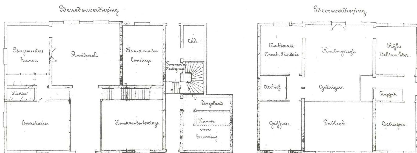
Afb. 3. Werktekening voor de verbouwing van het gemeentehuis in 1877.
