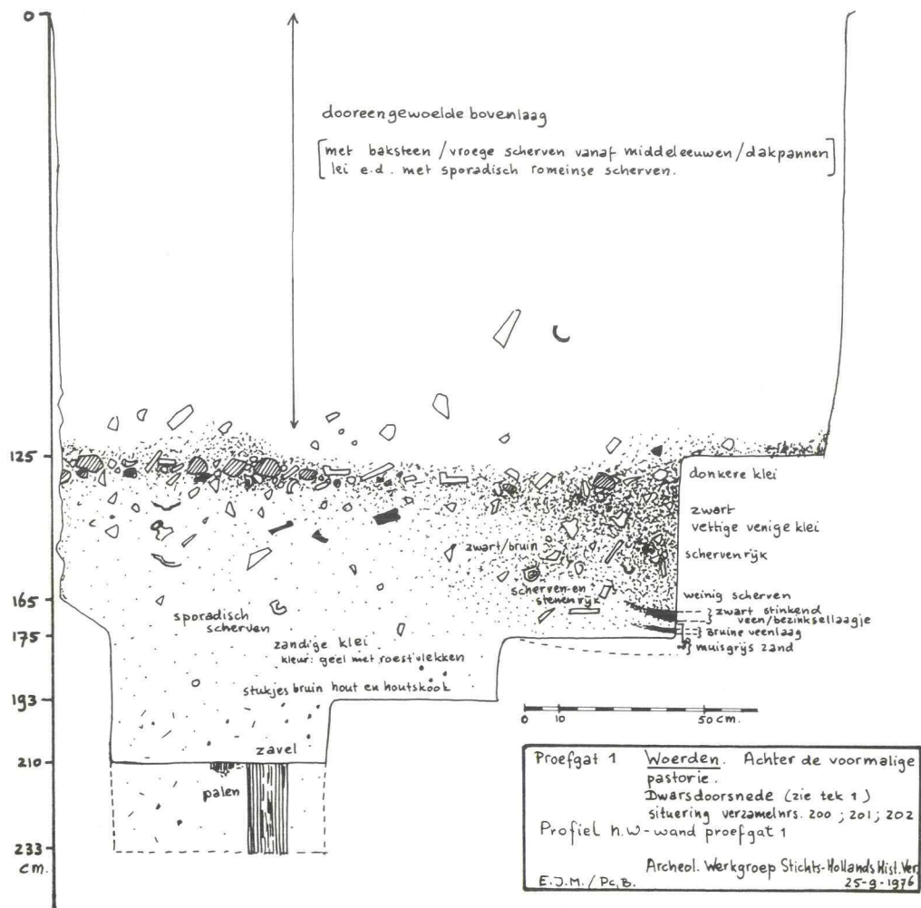
afb. 2 - Profieltekening noordwestelijke wand proefgat 1, E.J.M./Pc.B.
