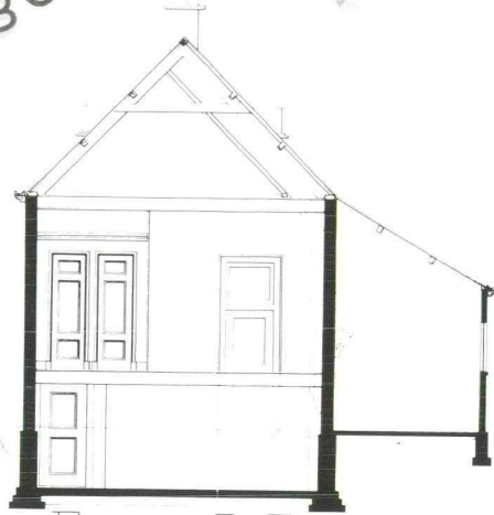
Doorsnede a-b
