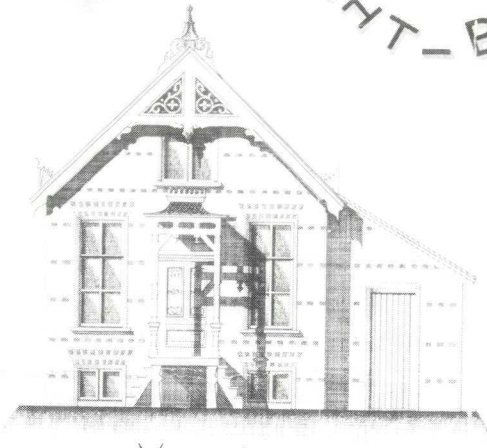
Voorgevel
