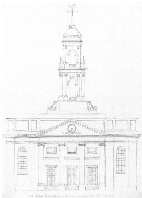
Grote Kerk te Hoorn, voorgevel van K.G. Zocher. Tekening door P. Jolly, 1852. Foto Rijksdienst Monumentenzorg Zeist.
