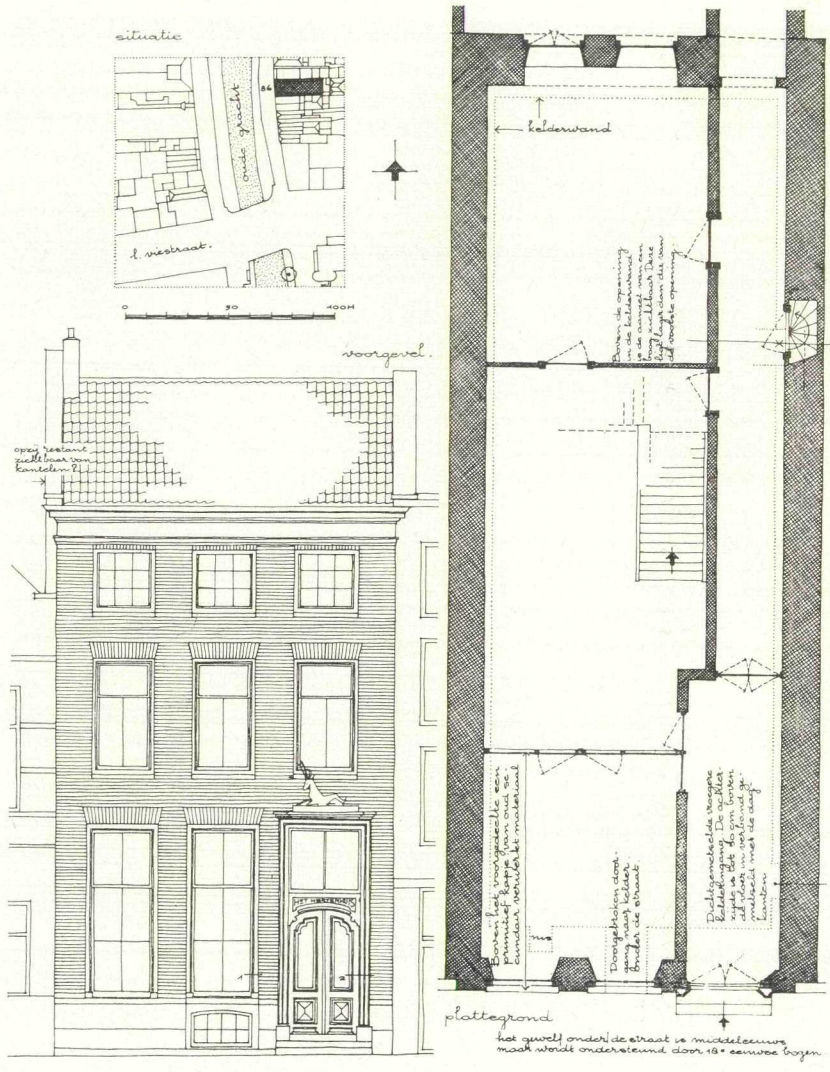
Afb. 1 (zie ook hiernaast). Het huis ten Hert, Oude Gracht 86.
