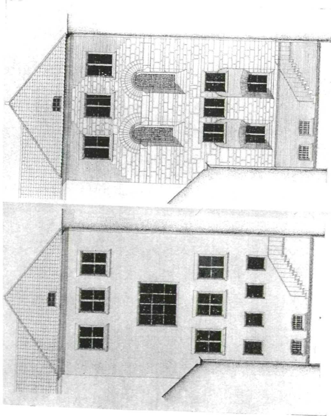
Zuidelijke transeptgevel der Sint Paulusabdij. Links zoals het plan voor de verbouwing was. Rechts hoe de gevel nu wordt.
