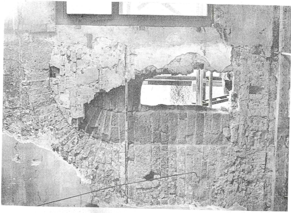
Westelijk venster in de zuidelijke transeptgevel (binnenzijde) van de Sint Paulusabdij komt tevoorschijn. Dit venster vindt men op het schetsplan terug en wel aan de buitenzijde rechts.
