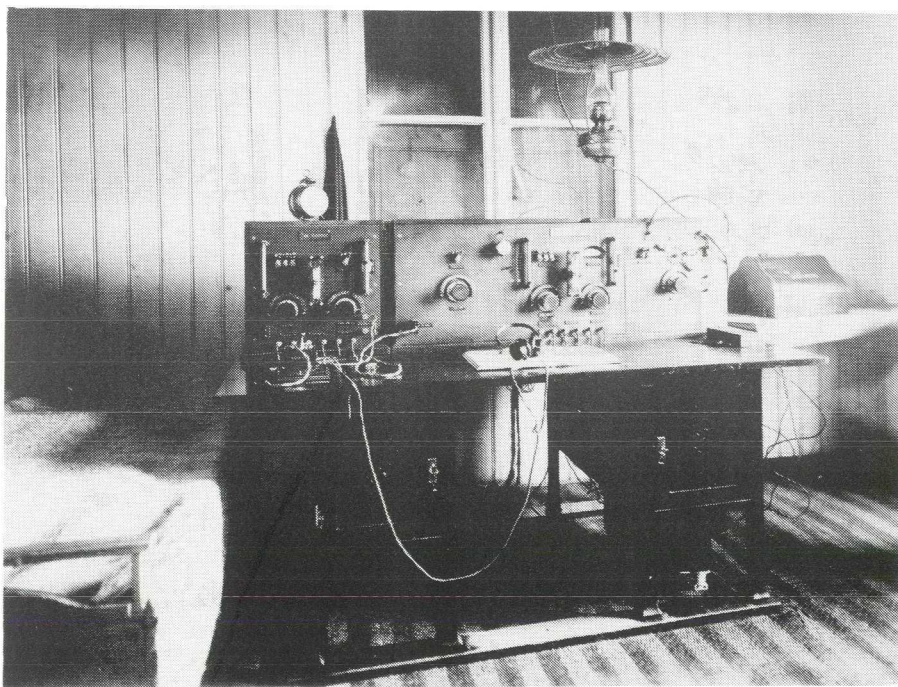
Het ontvangtoestel uit Indië (Philips Hilversum)
