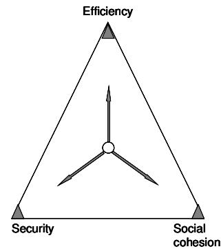
Trilemma
