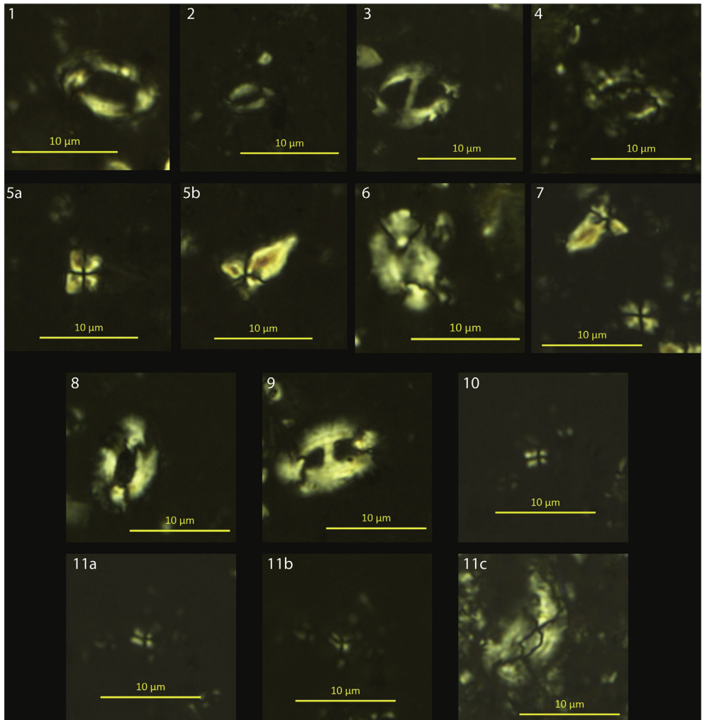
Fig. 4. Calcareous nannofossils. (1) Helicosphaera ampliaptera (sample CA10); (2) H. walbersdorfensis (sample CG13); (3) H. waltrans (sample CA20); (4) H. euphratis (sample CX14); (5a, b) Sphenolithus heteromorphus (sample CG1) at 0° and 45°; (6) S. heteromorphus and S. moriformis (sample BX13); (7) H. carteri (sample BX13); (8) H. intermedia (sample CA9); (9) H. ampliaptera (sample CA19); (10) H. mediterranea (sample CA20); (11a, b, c) S. disbelemnos (sample CA55) at 0°, 20° and 40°.
