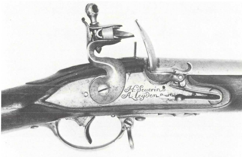
Het vuursteenslot als detail van het afgebeelde geweer.
